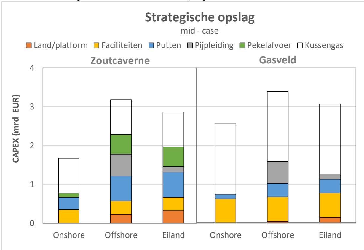
Figuur 5-4 Ingeschatte CAPEX investering voor strategische opslag (mid - case).
