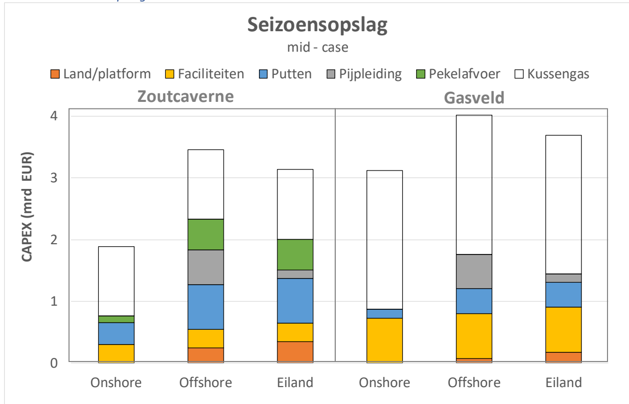
Figuur 5-3 Ingeschatte CAPEX-investering voor seizoensopslag (mid - case).
