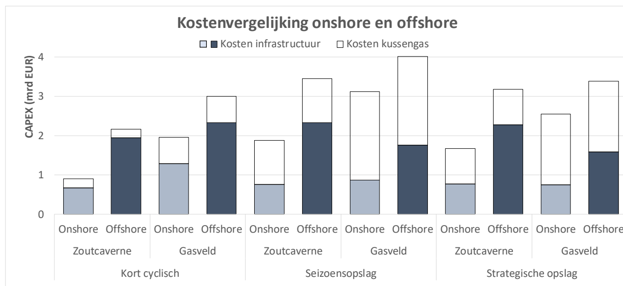
Figuur 5-5: Totale CAPEX kosten overzicht doorgerekend voor alle scenario's (mid-case).
