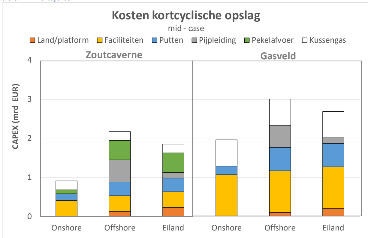
Figuur 5-2 Ingeschatte CAPEX investering voor kortcyclische opslag (mid-case).
