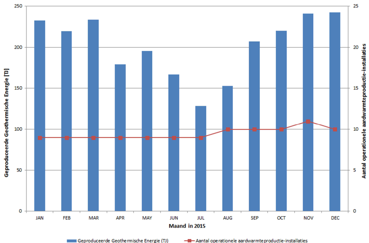
Figuur 16: Maandelijke productie aardwarmte of geothermische energie in Tera-Joules en het aantal aardwarmte productiesystemen dat heeft bijgedragen aan de gerapporteerde productie (exclusief Mijnwater energiecentrale Heerlen).
