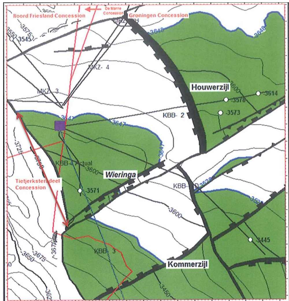
Figuur YYY.1 Structuurkaart en seismische doorsnede van het Wieringa veld (Winningplan Wieringa, NAM 2014). De diepte contourlijnen representeren de bovenkant van het Boven-Slochteren Zandsteen laagpakket.
