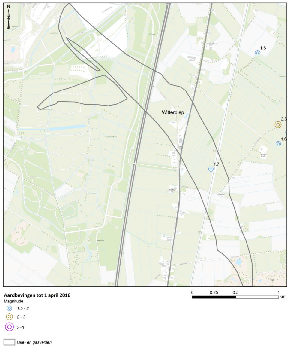
Figuur ZZZ.4 Geïnduceerde seismiciteit ( M_L \geq 1,5 ) voor het Witterdiep gasveld (zwarte contour).
