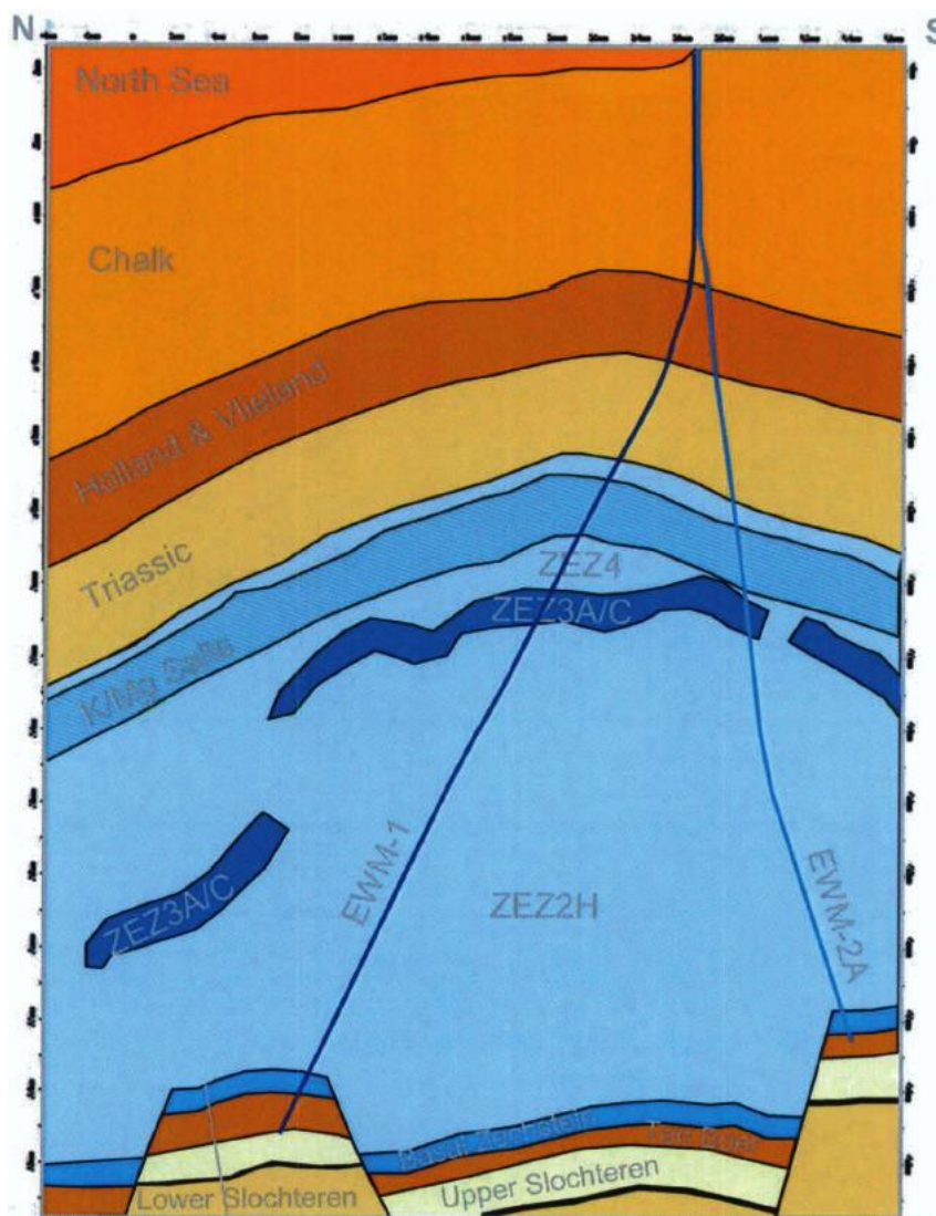
Figuur BBB.2 Doorsnede van het Oostrum veld (Winingsplan Kollum, NAM 2012).
