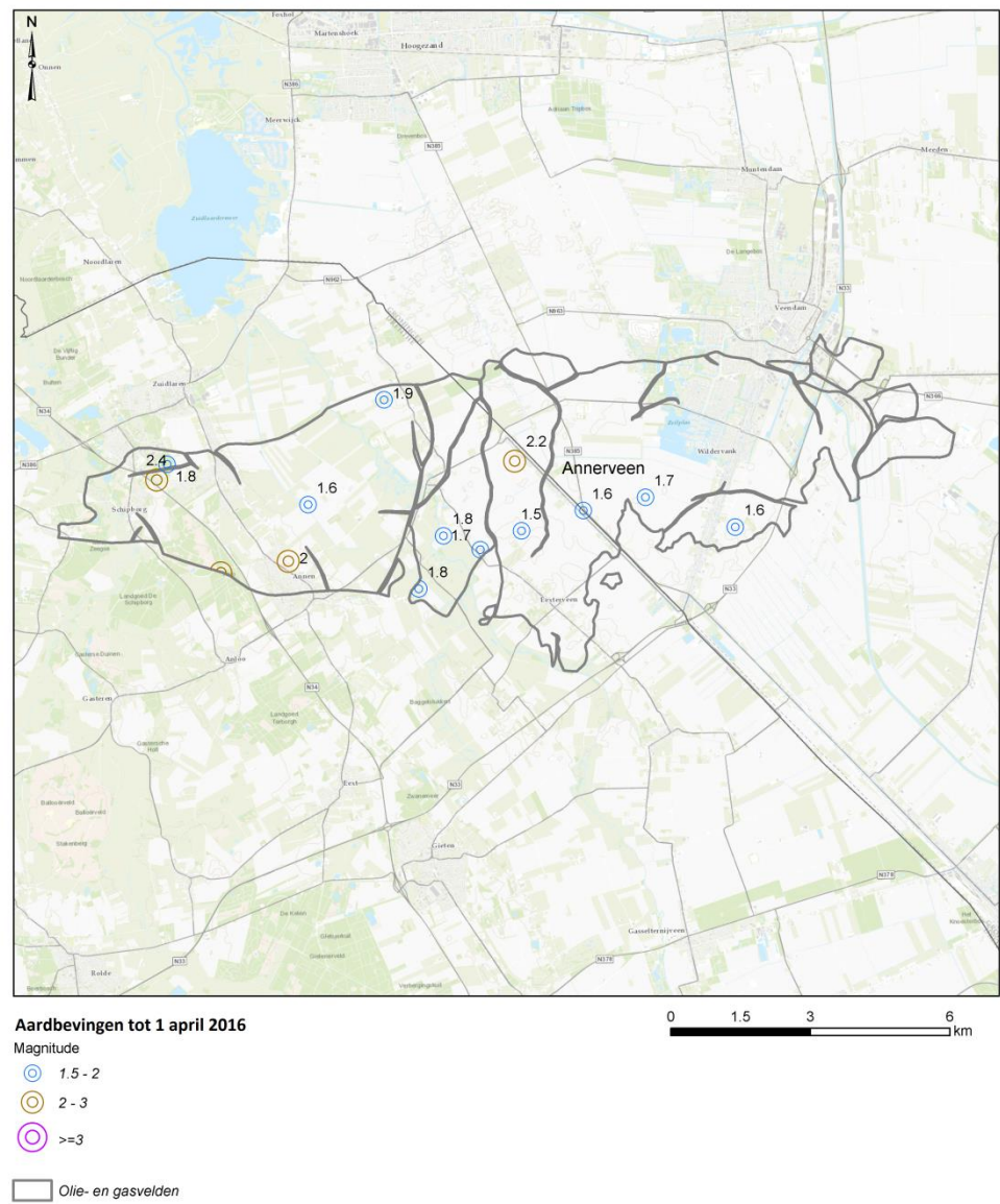
Figuur I.5 Geïnduceerde seismiciteit ( M_L \geq 1,5 ) voor het Annerveen gasveld.
