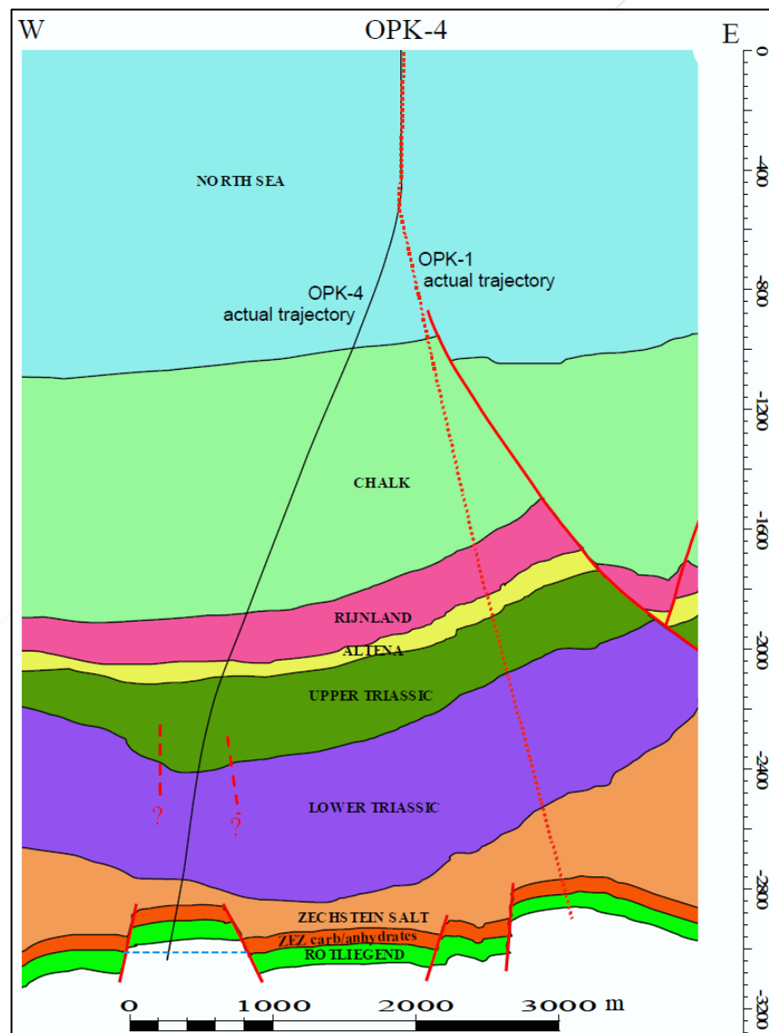
Figuur AAAA.2 Doorsnede van het gebied rondom het Zuidwending-Oost gasveld (Winningsplan Zuidwending-Oost, NAM 2006).
