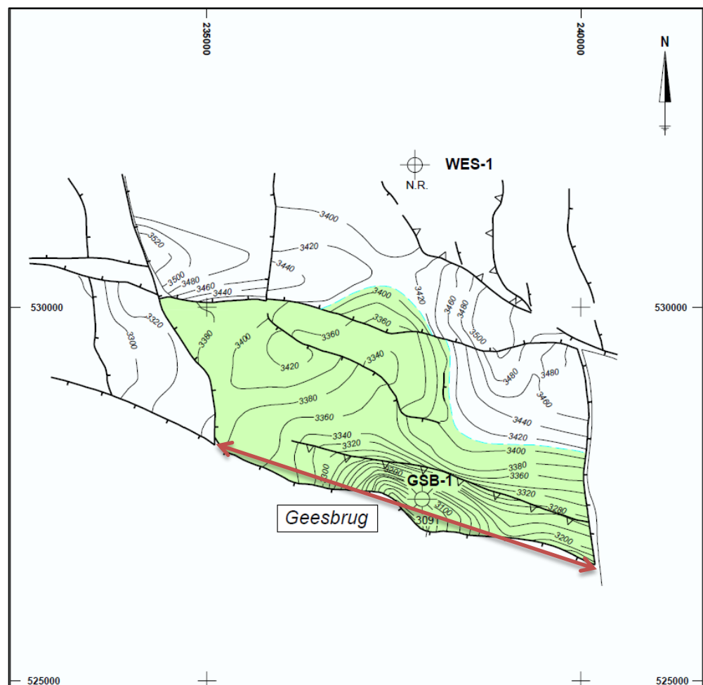
Figuur BB.1 Structuurkaart van het voorkomen in de Slochteren Formatie van het Geesbrug gasveld ( www.nlog.nl ). De diepte contourlijnen representeren de bovenkant van de Slochteren Formatie.
