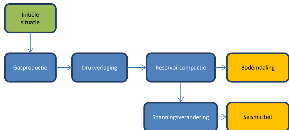
Figuur C.1. Schematische beschrijving van de relatie tussen gasproductie en de gevolgen voor bodemdaling en seismiciteit, waarop de gevolgd methode is afgestemd.
