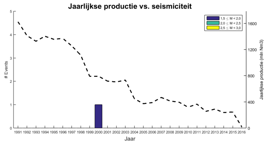
Figuur S.5 Geïnduceerde seismiciteit ( M_L \geq 1,5 ) voor het Coevorden gasveld in de tijd gerangschikt naar magnitude alsook de jaarlijkse productie (miljoen Nm 3 ).
