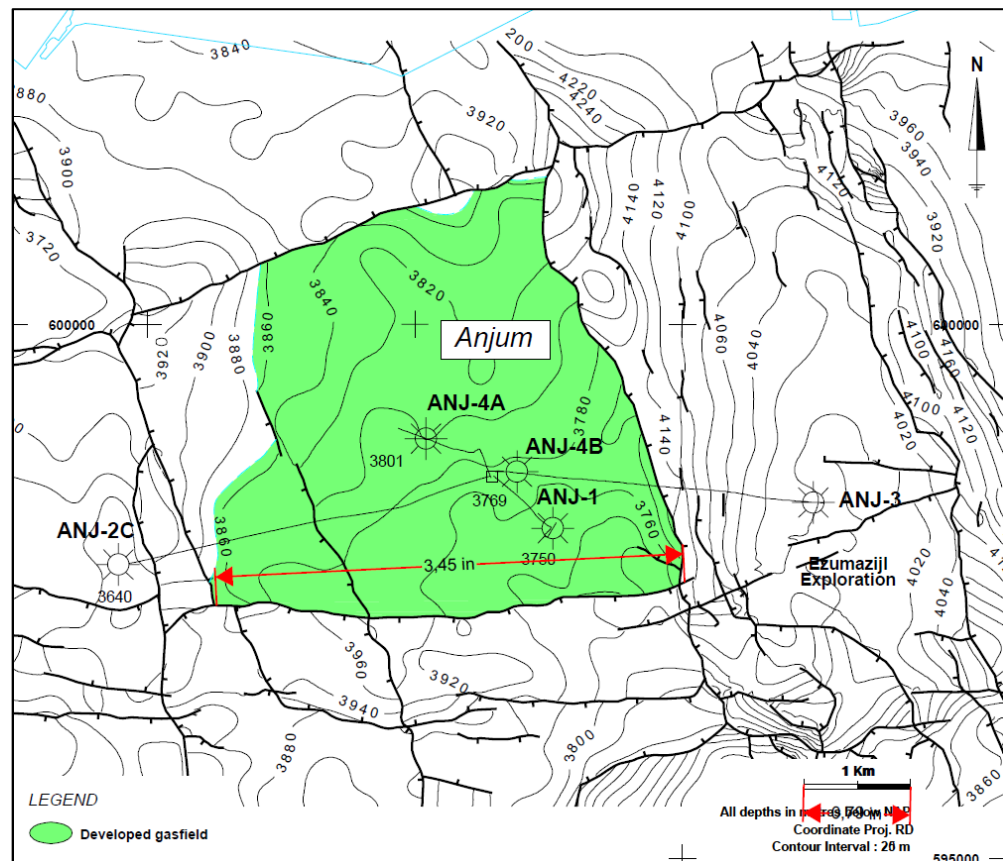
Figuur H.1 Structuurkaart van het Anjum gasveld (www.nlog.nl). De diepte contourlijnen representeren de bovenkant van de Boven-Rotliegend Groep. (De lengte van de breuk is gegeven in inch en is later omgerekend naar kilometers).
