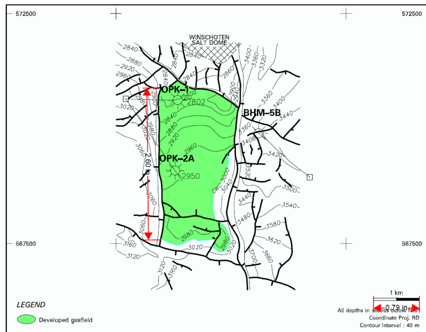
Figuur EEE.1 Structuurkaart van het Oude Pekela gasveld (www.nlog.nl). De diepte contourlijnen representeren de bovenkant van de Boven-Rotliegend Groep. (De lengte van de breuk is gegeven in inch en is later omgerekend naar kilometers).
