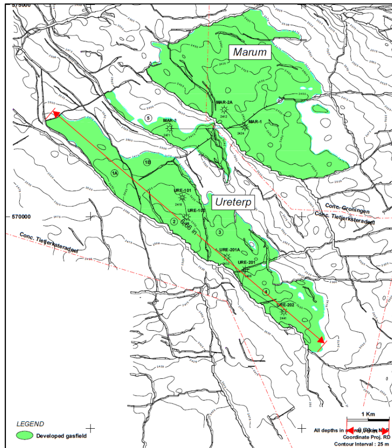
Figuur UUU.1 Structuurkaart van het Ureterp gasveld (www.nlog.nl). De diepte contourlijnen representeren de bovenkant van het Boven-Slochteren Laagpakket. (De lengte van de breuk is gegeven in inch en is later omgerekend naar kilometers).
