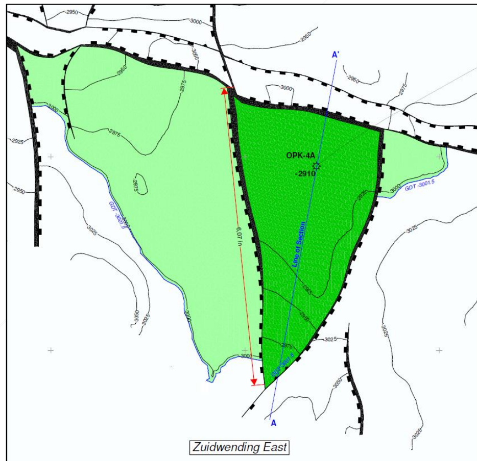
Figuur AAAA.1 Structuurkaart van het Zuidwending-Oost gasveld (Winningsplan Zuidwending-Oost, NAM 2011). De diepte contourlijnen representeren de bovenkant van de Boven-Rotliegend Groep. (De lengte van de breuk is gegeven in inch en is later omgerekend naar kilometers).
