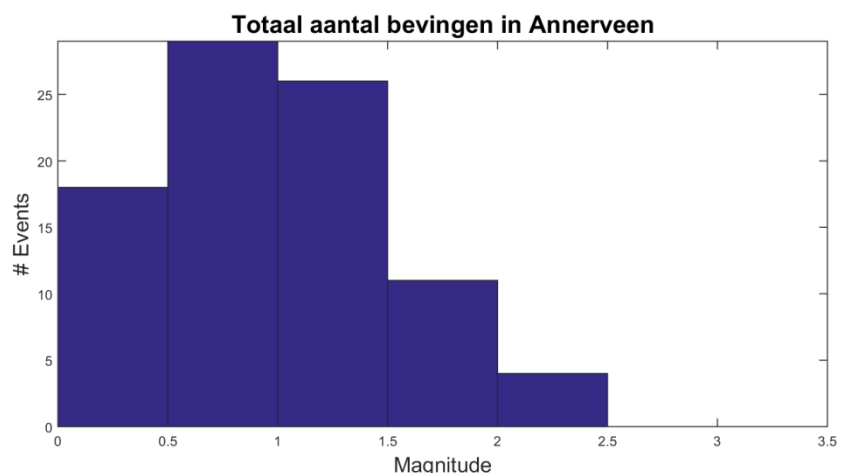
Figuur I.3 Histogram van de bevingen die in het Annerveen gasveld zijn opgetreden tot 01-04-2016.
