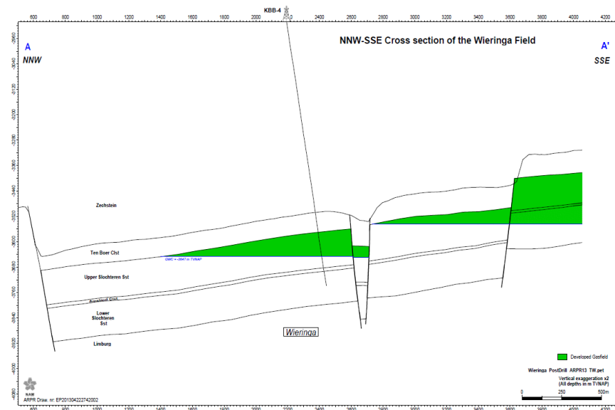
Figuur YYY.2 Geologische doorsnede van het Wieringa gasveld (Winingsplan Wieringa, NAM 2014).
