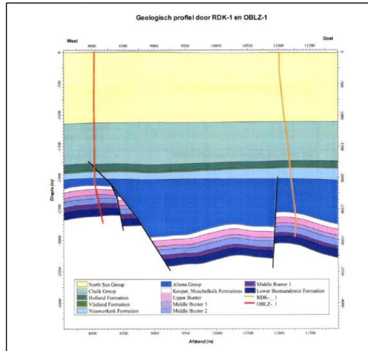
Figuur JJJ.2 Geologische doorsnede van de Reedijk en Oud-Beijerland Zuid gasvelden (Winingsplan Spijkenisse cluster, NAM 2003).
