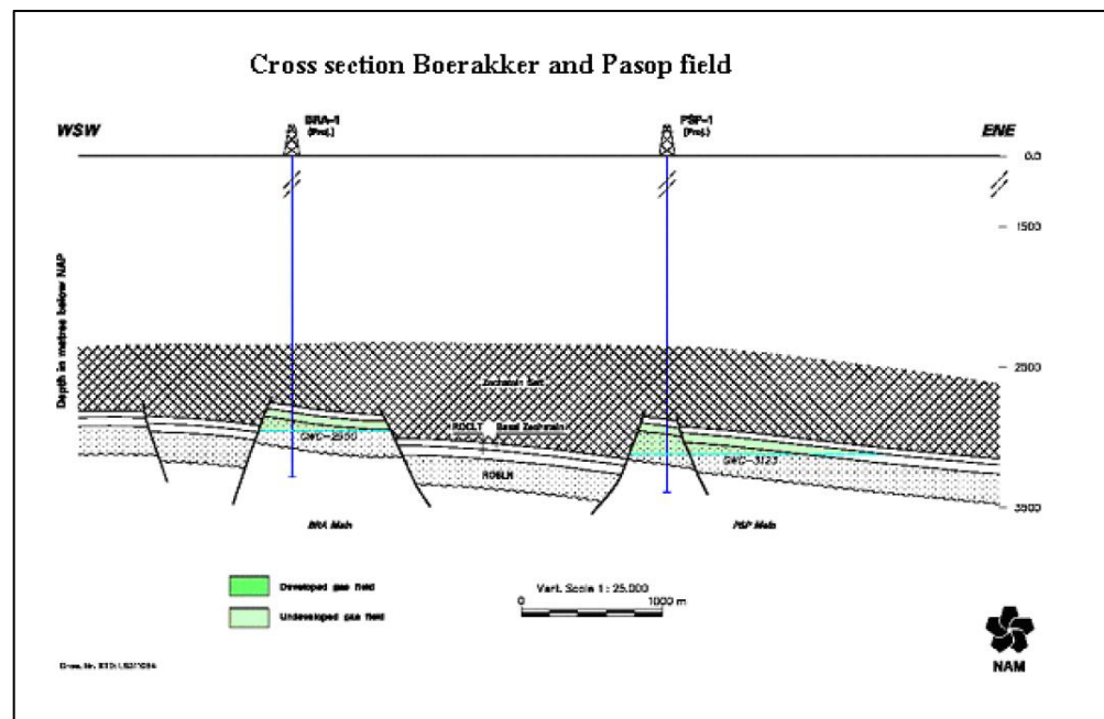
Figuur HHH.2 Geologische doorsnede van het Pasop en Boerakker gasveld (Winningsplan Grijpskerk-Zuid, NAM 2005).
