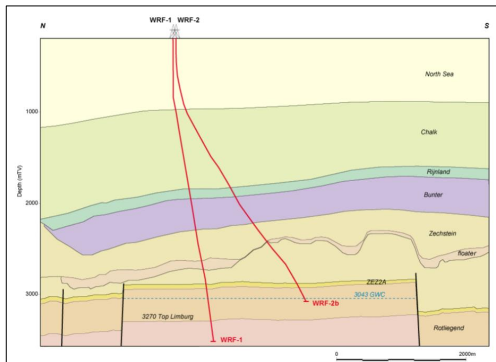
Figuur XXX.2 Doorsnede van het Warffum gasveld (uit: Winningsplan 2003 van de NAM).
