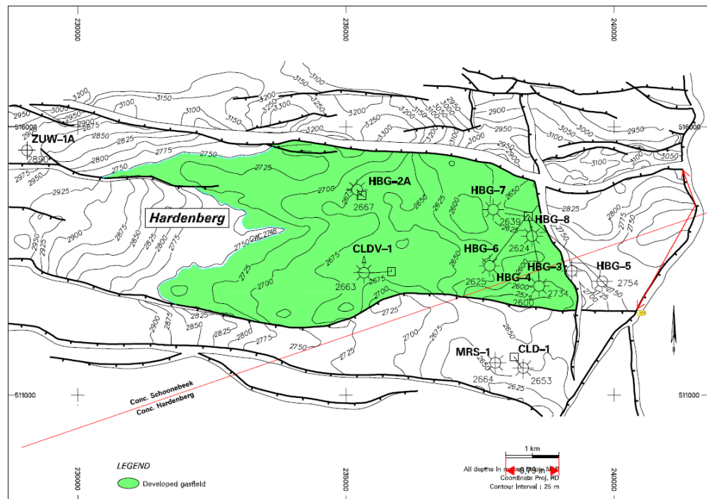
Figuur GG.1 Structuurkaart van het Hardenberg (groen) en Hardenberg-Oost gasveld (breukblokken ten oosten van Hardenberg veld) ( www.nlog.nl ). De diepte contourlijnen representeren de bovenkant van de Limburg Groep. (De lengte van de breuk is gegeven in inch en is later omgerekend naar kilometers).
