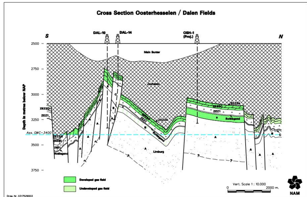
Figuur U.3 Doorsnede van de Dalen en Oosterhesselen gasvelden (Winningplan zuidoost Drenthe Zuur, NAM 2005).
