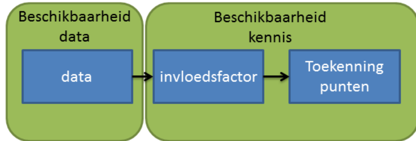
Figuur 5-1. Schema van toekenning score in de seismische risicoanalyse (SRA) en de benodigde informatie voor de elementen.
