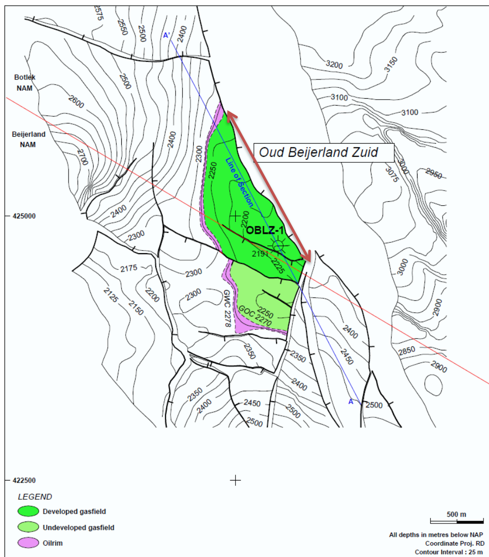
Figuur DDD.1 Structuurkaart van het Röt voorkomen van het Oud-Beijerland Zuid gasveld (www.nlog.nl). De diepte contoulijnien representeren de top van de Röt Formatie.
